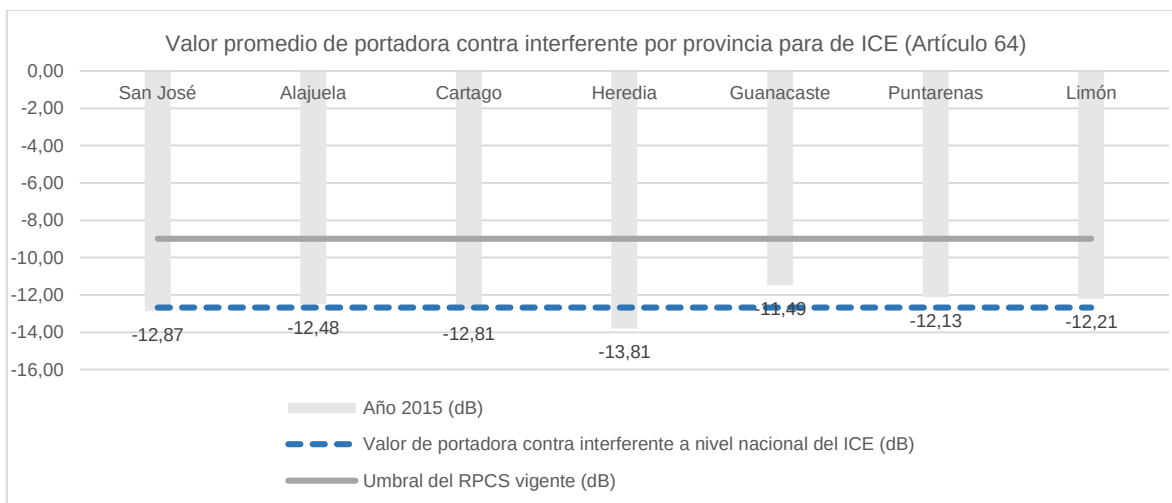
Figura 9. Valor promedio de portadora contra interferente por provincia para el operador ICE, así como el valor promedio a nivel nacional y su contraste contra el umbral establecido en el RPCS vigente.
