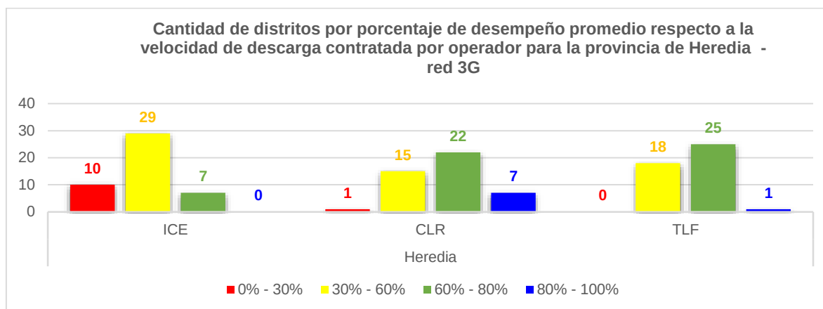
Figura 41. Cantidad de distritos por porcentaje de desempeño promedio respecto a la velocidad de descarga contratada para los operadores ICE, CLR y TLF en la provincia de Heredia para la red 3G 12 .
