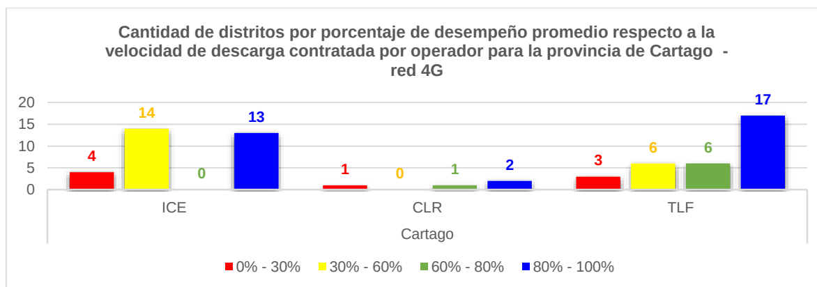
Figura 47. Cantidad de distritos por porcentaje de desempeño promedio respecto a la velocidad de descarga contratada para los operadores ICE, CLR y TLF en la provincia de Cartago para la red 4G 18 .
