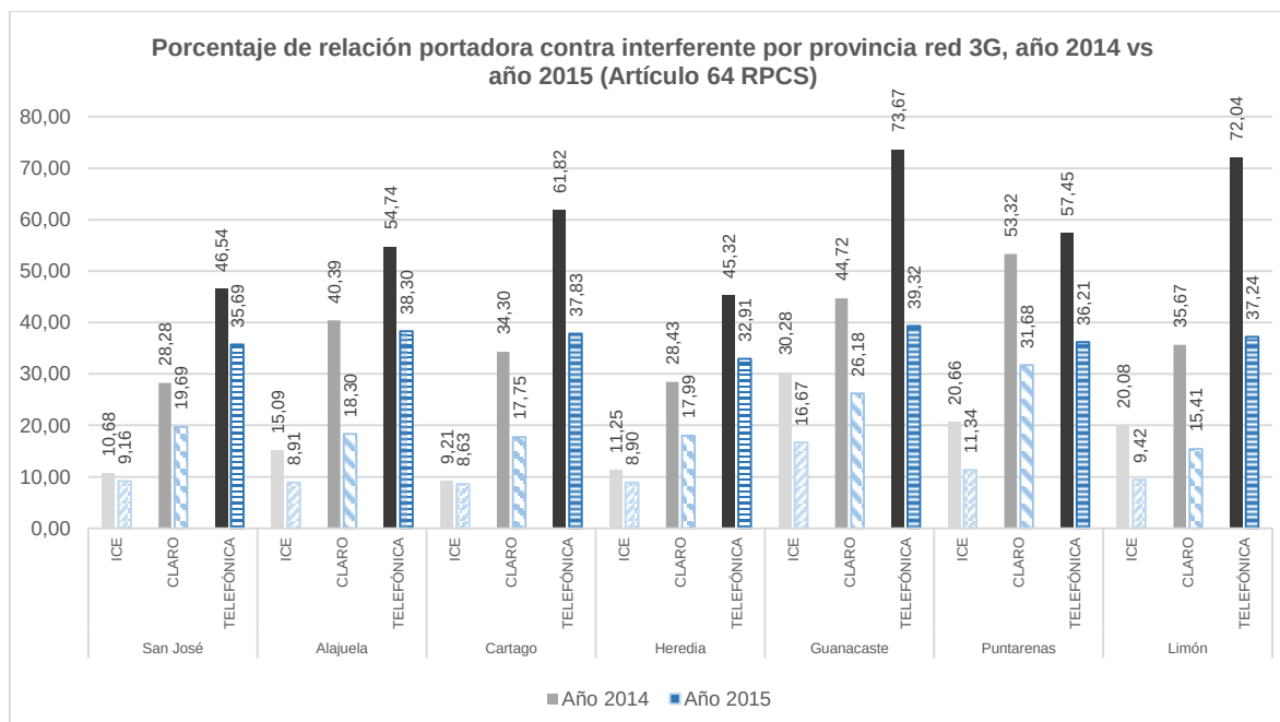
Figura 8. Resultados de portadora contra interferente detallado por provincia para la Red 3G del ICE, CLR y TLF, año 2014 (escala grises) respecto al año 2015 (escala azules con trama).
