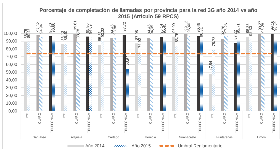
Figura 3. Resultados de porcentaje de completación de llamadas por provincia para la red 3G de los operadores ICE, CLR y TLF, año 2014 (escala grises) respecto al año 2015 (escala azules con trama).
