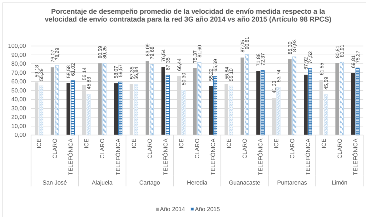
Figura 30. Resultados del porcentaje promedio de desempeño de envío de datos detallado por provincia para la Red 3G del ICE, CLR y TLF, año 2014 (escala grises) respecto al año 2015 (escala azules con trama).
