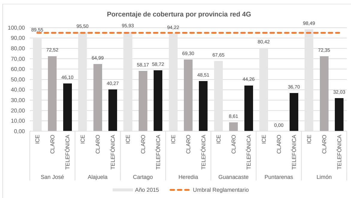
Figura 7. Resultados de porcentaje de cobertura detallado por provincia para la Red 4G de los operadores ICE, CLR y TLF 7 .
