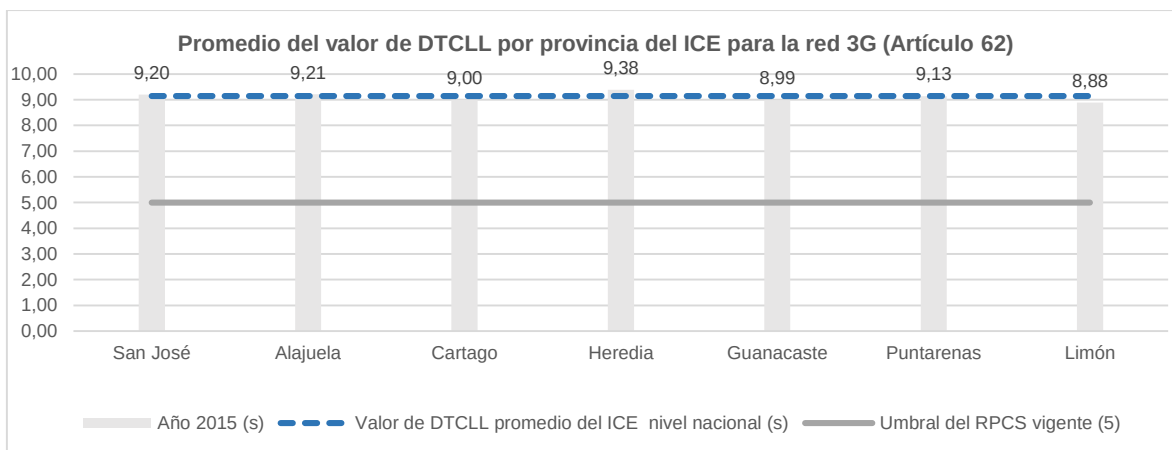
Figura 17. Valor promedio de DTCLL por provincia para la red 3G para el operador ICE, así como el valor promedio a nivel nacional y su contraste contra el umbral establecido en el RPCS vigente.
