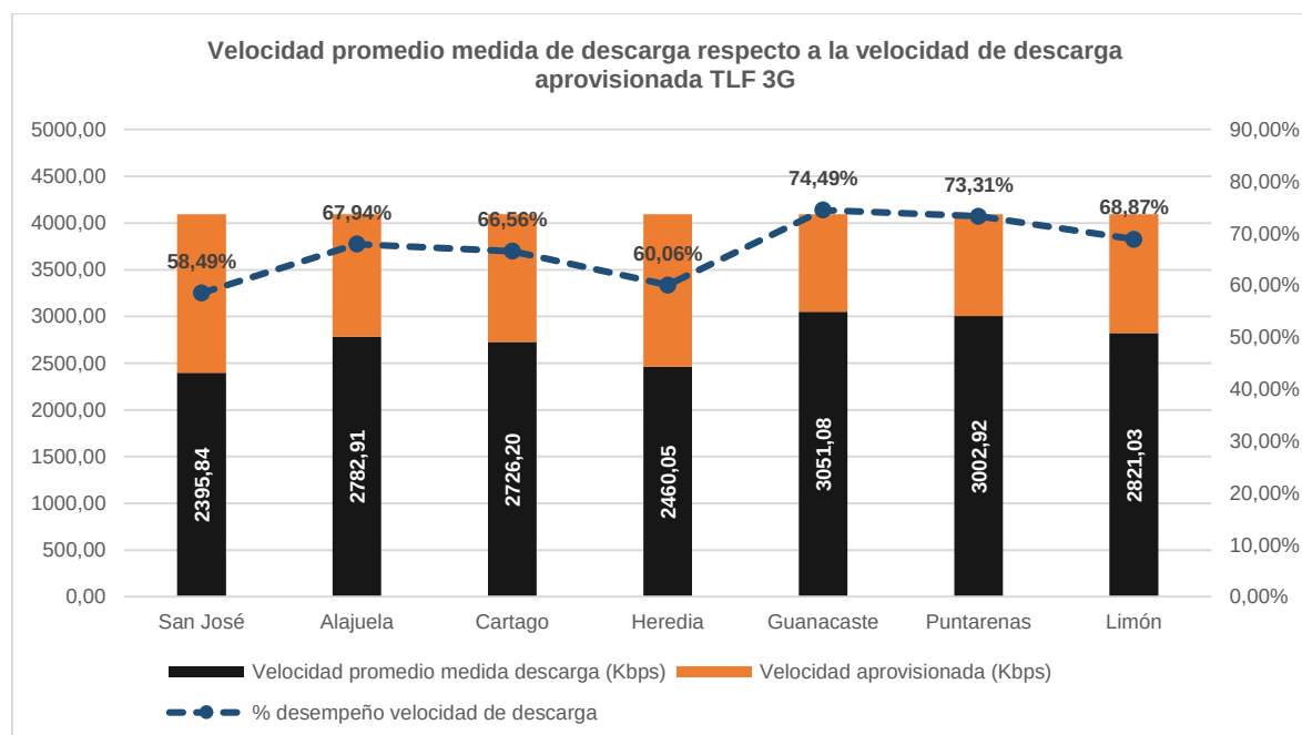
Figura 25. Valor promedio de velocidad de descarga por provincia para el operador TLF, así como el valor de velocidad aprovisionada (ambos eje de la izquierda), respecto al porcentaje de desempeño de velocidad de descarga (eje de la derecha), para la red 3G.
