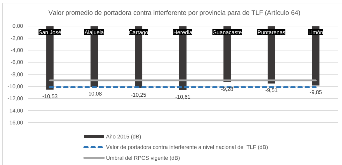
Figura 11. Valor promedio de portadora contra interferente por provincia para el operador TLF, así como el valor promedio a nivel nacional y su contraste contra el umbral establecido en el RPCS vigente.
