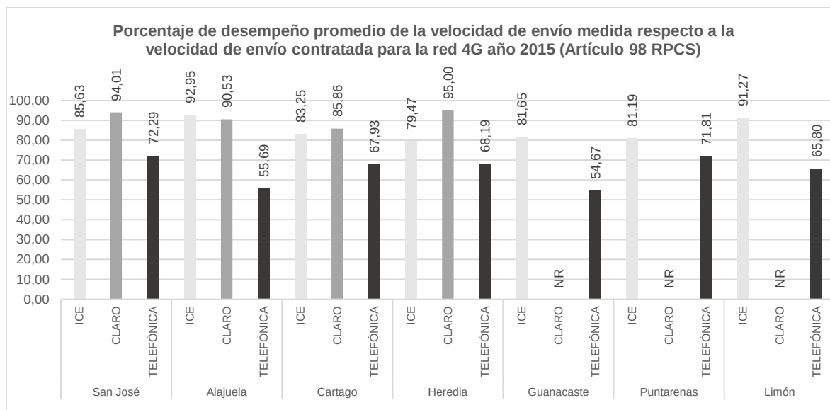
Figura 34. Resultados del porcentaje promedio de desempeño de envío de datos detallado por provincia para la red 4G del ICE, CLR y TLF, año 2015.
