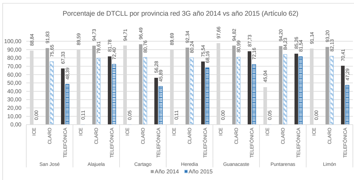
Figura 16. Resultados de DTCLL detallado por provincia para la Red 3G del ICE, CLR y TLF, año 2014 (escala grises) respecto al año 2015 (escala azules con trama).
