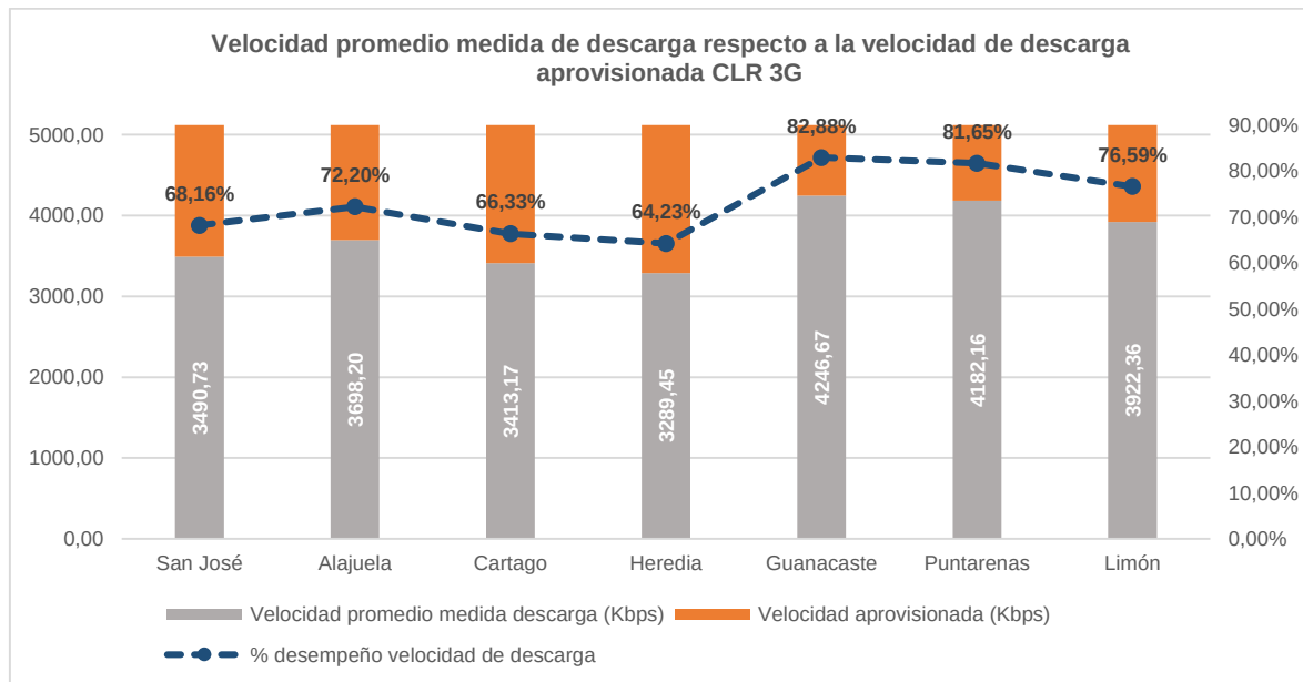
Figura 24. Valor promedio de velocidad de descarga por provincia para el operador CLR, así como el valor de velocidad aprovisionada (ambos eje de la izquierda), respecto al porcentaje de desempeño de velocidad de descarga (eje de la derecha), para la red 3G.
