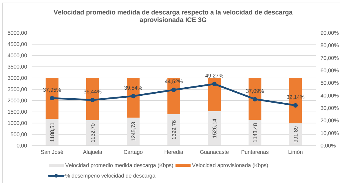
Figura 23. Valor promedio de velocidad de descarga por provincia para el operador ICE, así como el valor de velocidad aprovisionada (ambos eje de la izquierda), respecto al porcentaje de desempeño de velocidad de descarga (eje de la derecha), para la red 3G.
