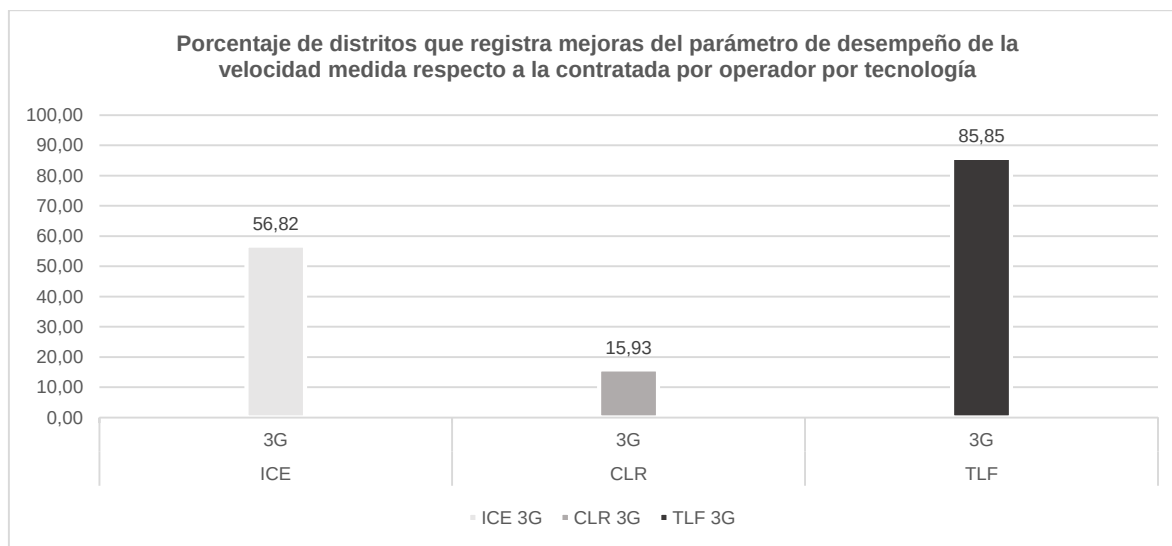
Figura 57. Porcentaje de distritos que registran mejoras del parámetro de porcentaje de desempeño por operador y tecnología, generado a partir de la comparativa del año 2014 respecto al año 2015.
