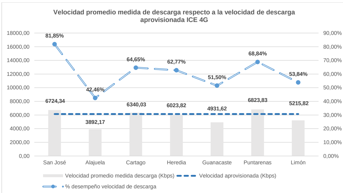
Figura 27. Valor promedio de velocidad de descarga por provincia para el operador ICE, así como el valor de velocidad aprovisionada (ambos eje de la izquierda), respecto al porcentaje de desempeño de velocidad de descarga (eje de la derecha), para la red 4G.
