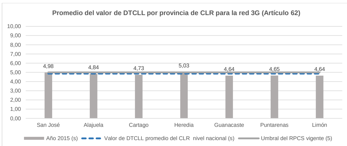
Figura 18. Valor promedio de DTCLL por provincia para la red 3G para el operador CLR, así como el valor promedio a nivel nacional y su contraste contra el umbral establecido en el RPCS vigente.
