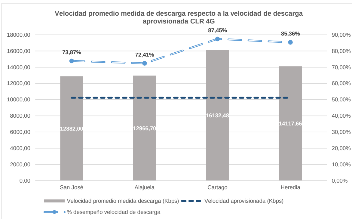
Figura 28. Valor promedio de velocidad de descarga por provincia para el operador CLR, así como el valor de velocidad aprovisionada (ambos eje de la izquierda), respecto al porcentaje de desempeño de velocidad de descarga (eje de la derecha), para la red 4G.
