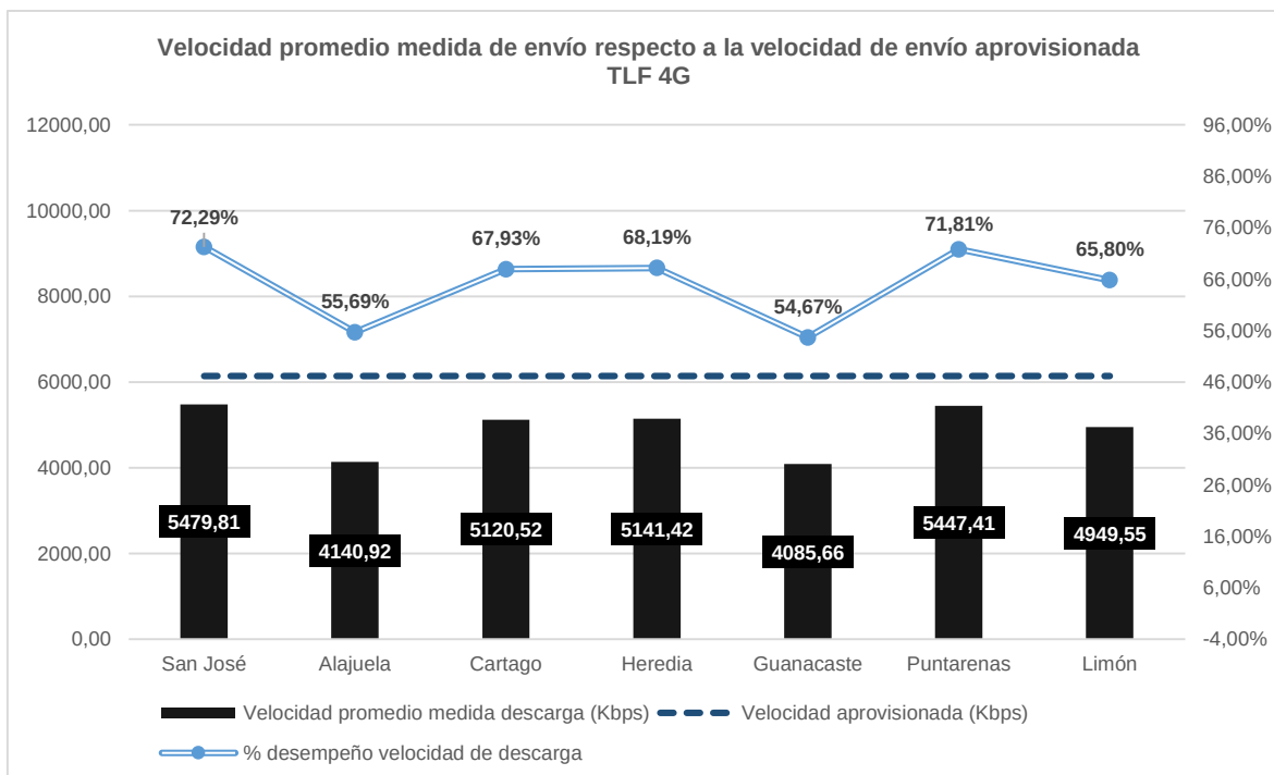
Figura 37. Valor promedio de velocidad de envío por provincia para el operador TLF, así como el valor de velocidad aprovisionada (ambos eje de la izquierda), respecto al porcentaje de desempeño de velocidad de envío (eje de la derecha), para la red 4G.
