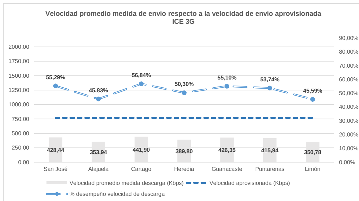
Figura 31. Valor promedio de velocidad de envío por provincia para el operador ICE, así como el valor de velocidad aprovisionada (ambos eje de la izquierda), respecto al porcentaje de desempeño de velocidad de envío (eje de la derecha), para la red 3G.
