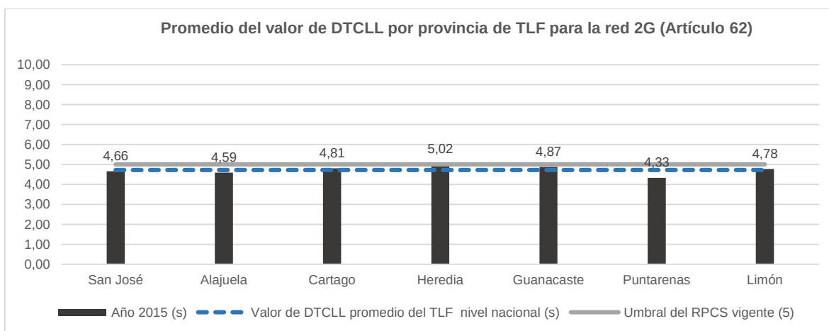
Figura 15. Valor promedio de DTCLL por provincia para la red 2G para el operador TLF, así como el valor promedio a nivel nacional y su contraste contra el umbral establecido en el RPCS vigente.
