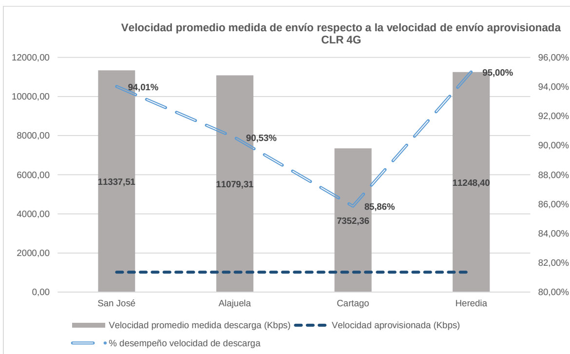
Figura 36. Valor promedio de velocidad de envío por provincia para el operador CLR, así como el valor de velocidad aprovisionada (ambos eje de la izquierda), respecto al porcentaje de desempeño de velocidad de envío (eje de la derecha), para la red 4G.
