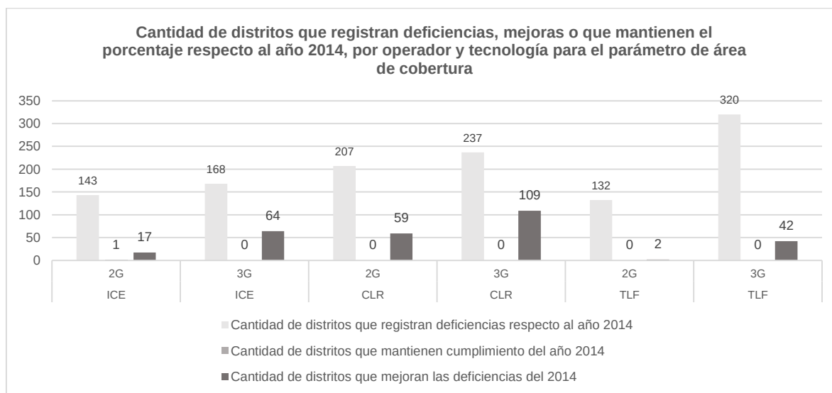
Figura 52. Cantidad de distritos que registran mejoras respecto al año 2014, cantidad de distritos que registran deficiencias superiores a las registradas en el 2014 y cantidad de distritos que mantiene el porcentaje de área de cobertura.
