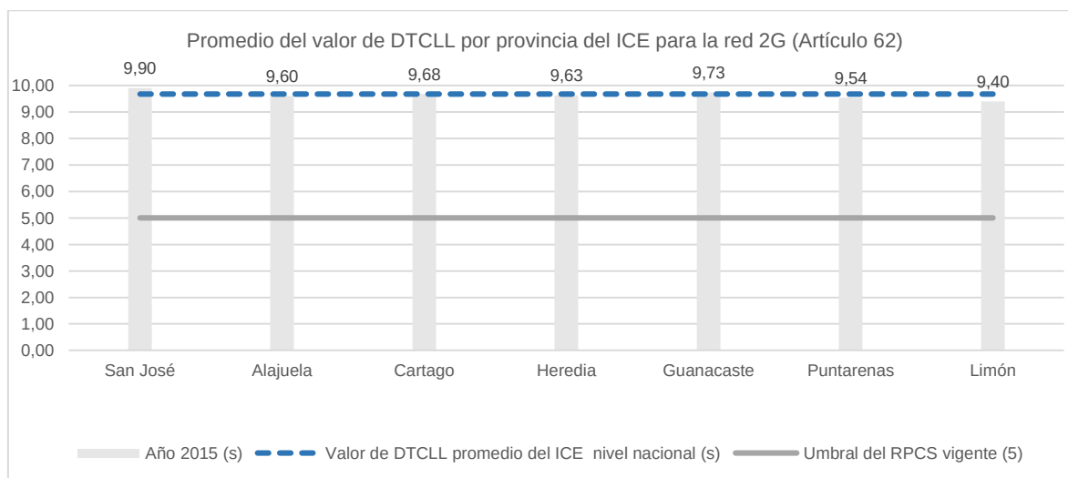
Figura 13. Valor promedio de DTCLL por provincia para la red 2G para el operador ICE, así como el valor promedio a nivel nacional y su contraste contra el umbral establecido en el RPCS vigente.
