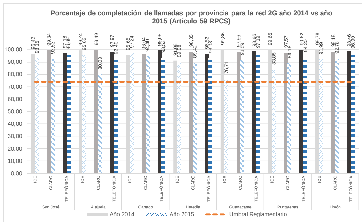
Figura 2. Resultados de porcentaje de completación de llamadas por provincia para la red 2G de los operadores ICE, CLR y TLF, año 2014 (escala grises) vs año 2015 (escala azules con trama).
