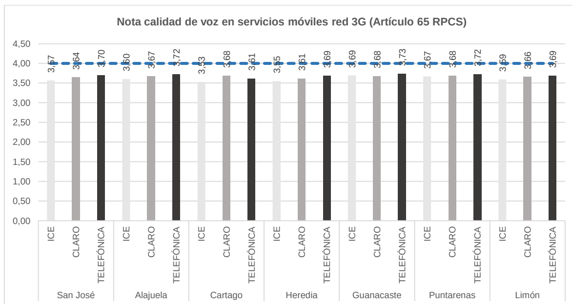
Figura 21. Nota de calidad de voz detallado por provincia para la Red 3G del ICE, CLR y TLF, año 2015.
