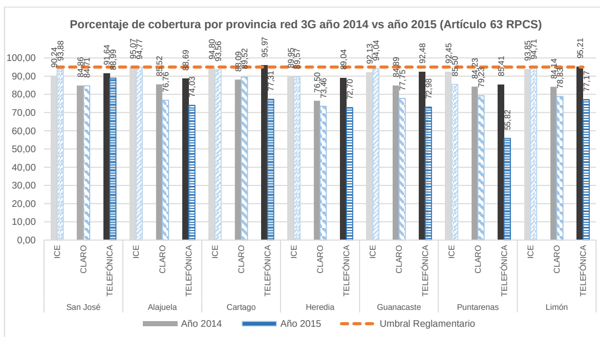
Figura 6. Resultados de porcentaje de cobertura detallado por provincia para la Red 3G de los operadores ICE, CLR y TLF, año 2014 (escala grises) respecto al año 2015 (escala azules con trama).
