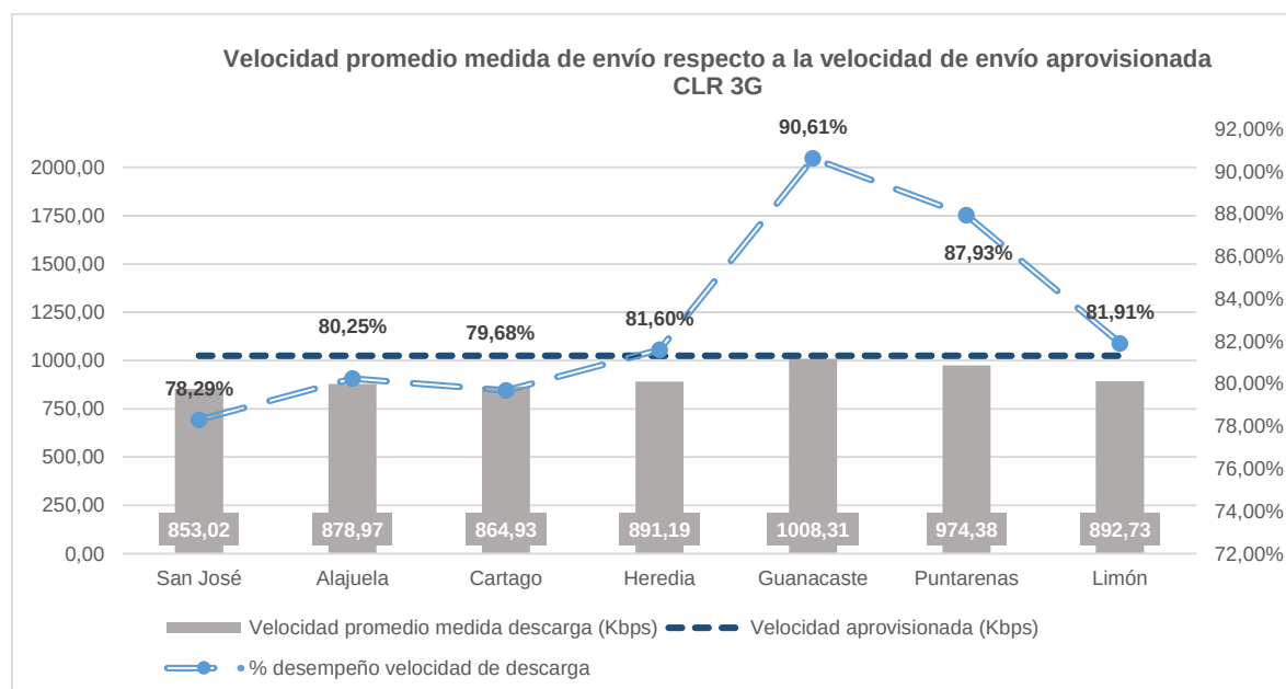
Figura 32. Valor promedio de velocidad de envío por provincia para el operador CLR, así como el valor de velocidad aprovisionada (ambos eje de la izquierda), respecto al porcentaje de desempeño de velocidad de envío (eje de la derecha), para la red 3G.
