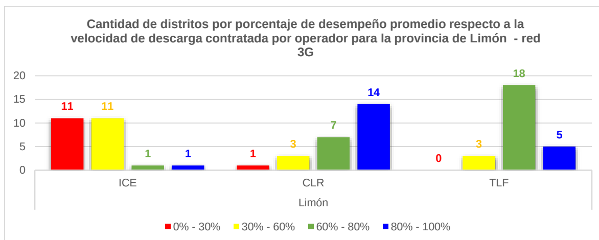
Figura 44. Cantidad de distritos por porcentaje de desempeño promedio respecto a la velocidad de descarga contratada para los operadores ICE, CLR y TLF en la provincia de Limón para la red 3G 15 .
