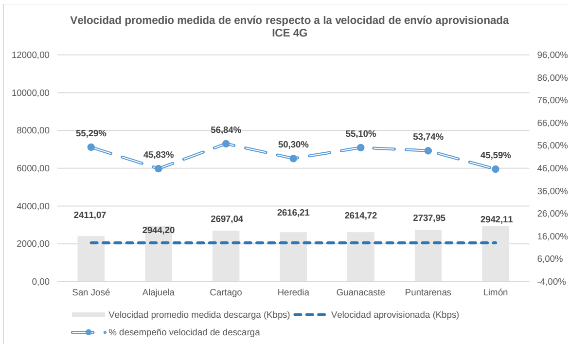
Figura 35. Valor promedio de velocidad de envío por provincia para el operador ICE, así como el valor de velocidad aprovisionada (ambos eje de la izquierda), respecto al porcentaje de desempeño de velocidad de envío (eje de la derecha), para la red 4G.
