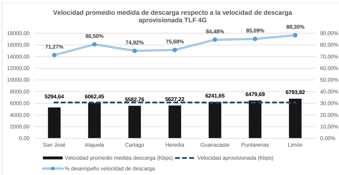
Figura 29. Valor promedio de velocidad de descarga por provincia para el operador TLF, así como el valor de velocidad aprovisionada (ambos eje de la izquierda), respecto al porcentaje de desempeño de velocidad de descarga (eje de la derecha), para la red 4G.
