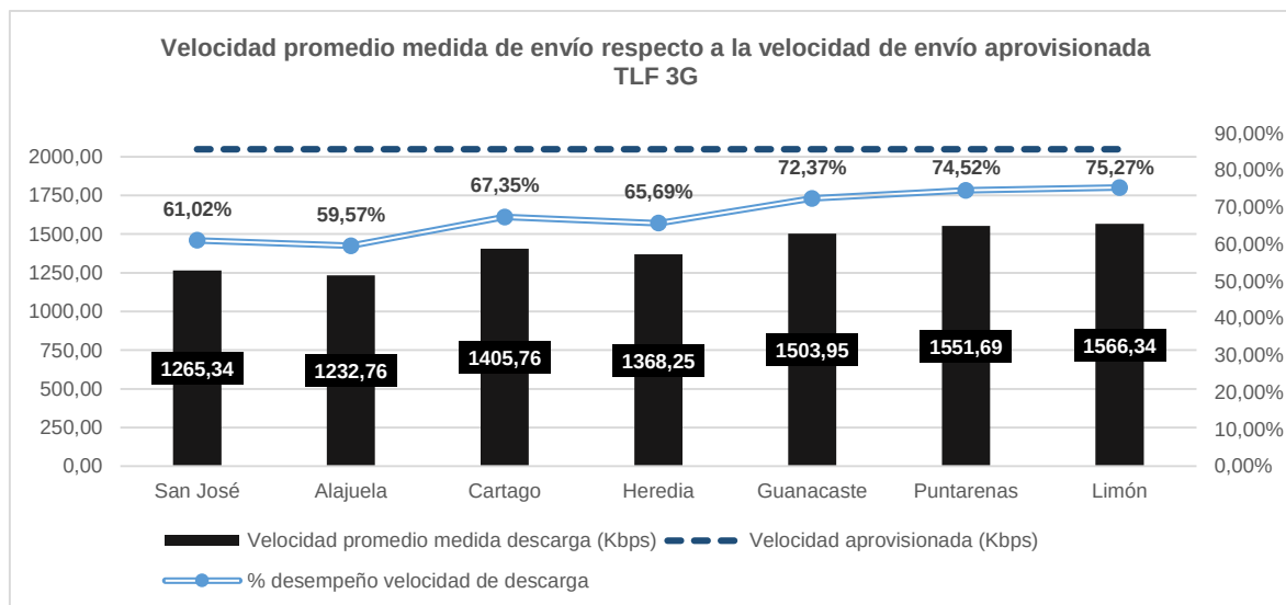
Figura 33. Valor promedio de velocidad de envío por provincia para el operador TLF, así como el valor de velocidad aprovisionada (ambos eje de la izquierda), respecto al porcentaje de desempeño de velocidad de envío (eje de la derecha), para la red 3G.
