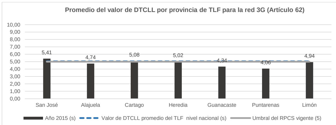
Figura 19. Valor promedio de DTCLL por provincia para la red 3G para el operador TLF, así como el valor promedio a nivel nacional y su contraste contra el umbral establecido en el RPCS vigente.
