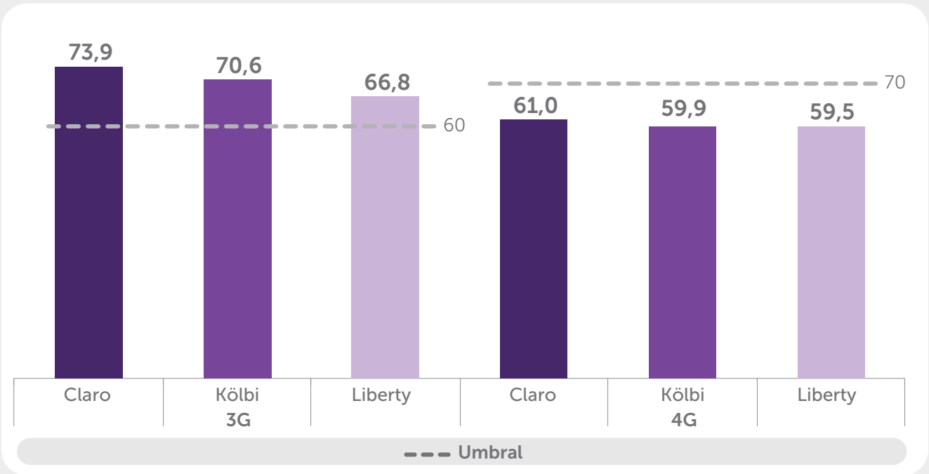
GRÁFICO 13. Mediciones respecto de la velocidad de descarga promedio en las redes 3G y 4G, 2025 (Cifras en porcentajes)
