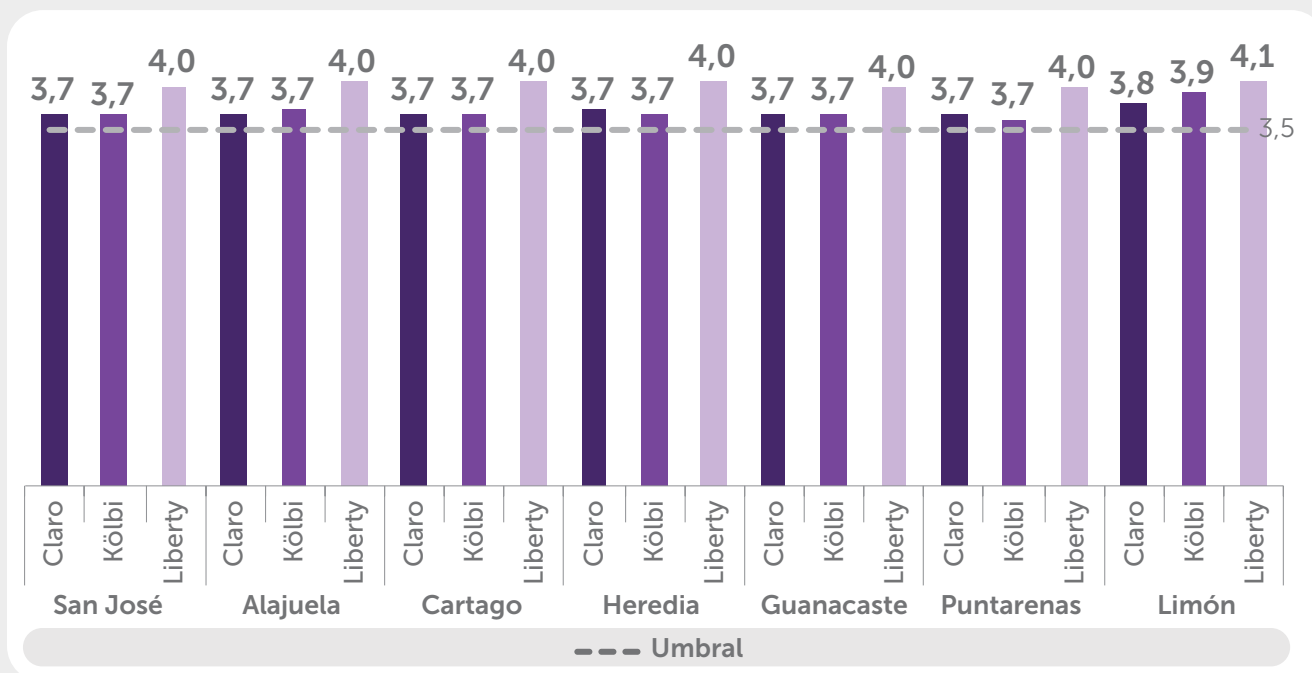
GRÁFICO 9. Resultados de calidad de voz en la red 3G por provincia, para el año 2025 (Cifras en porcentajes)
