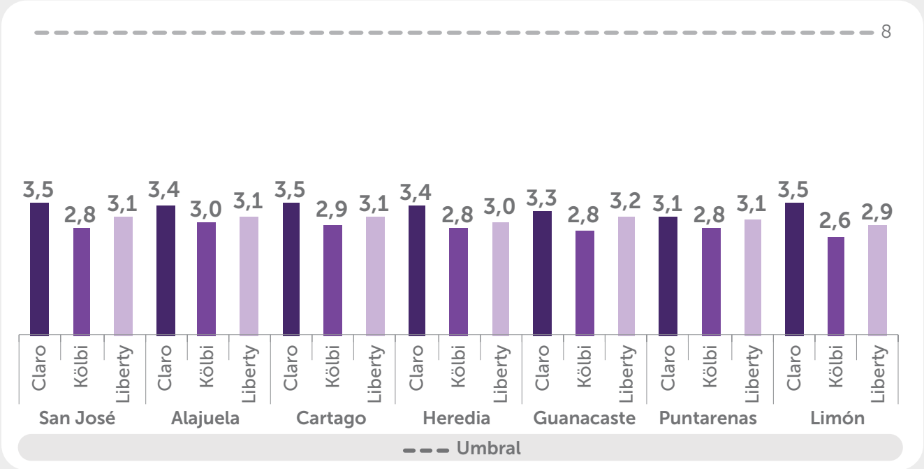
GRÁFICO 7. Tiempo de establecimiento de llamada en la red 3G por provincia, para el año 2025
