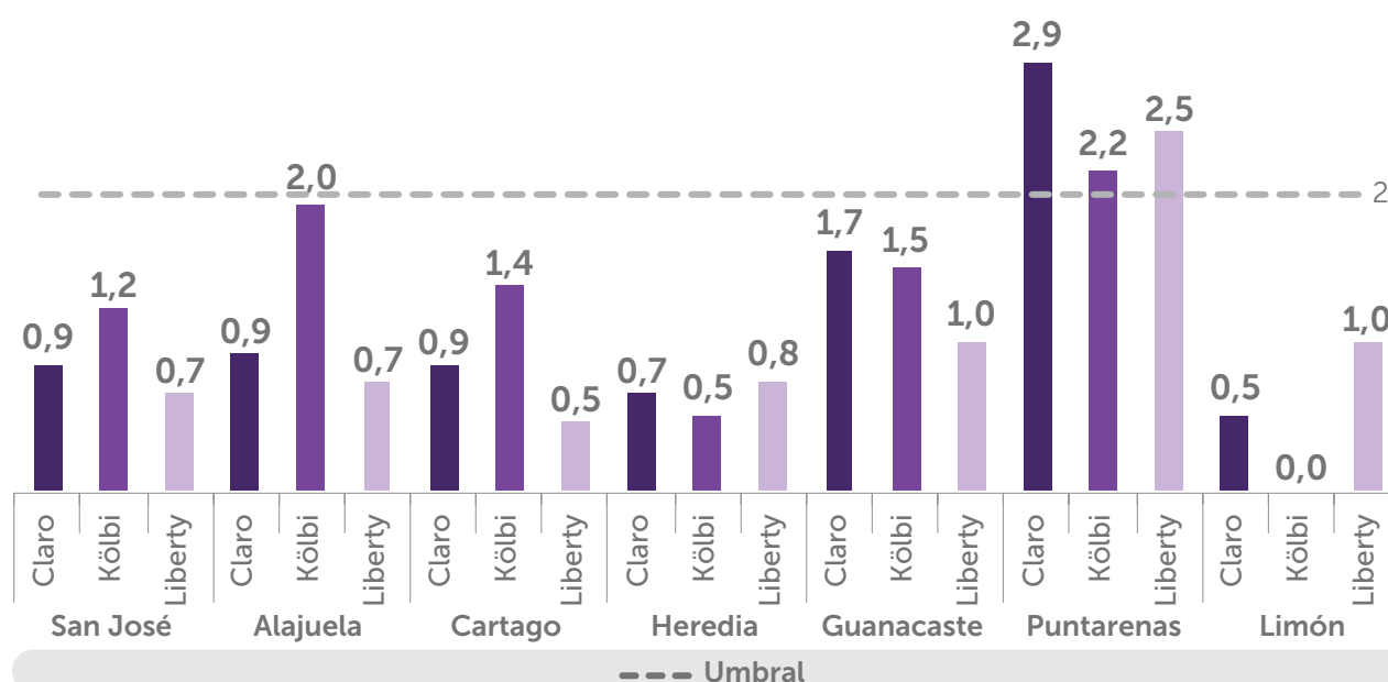
GRÁFICO 5. Porcentaje de llamadas interrumpidas en la red 3G por provincia, para el año 2025 (Cifras en porcentajes)
