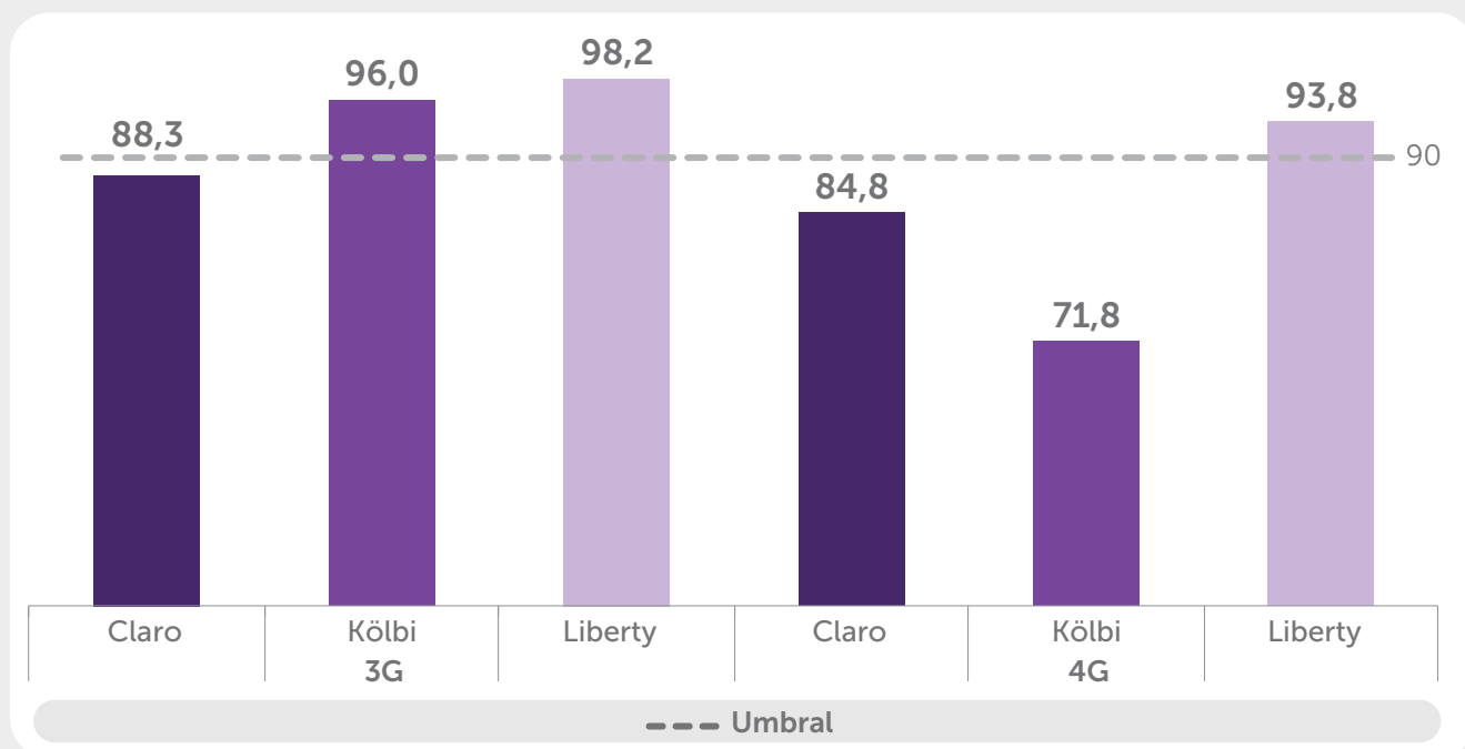
GRÁFICO 1. Precisión de cobertura para las redes 3G y 4G en 2025, porcentaje de muestras que cumplen con el área de cobertura (Cifras en porcentajes)
