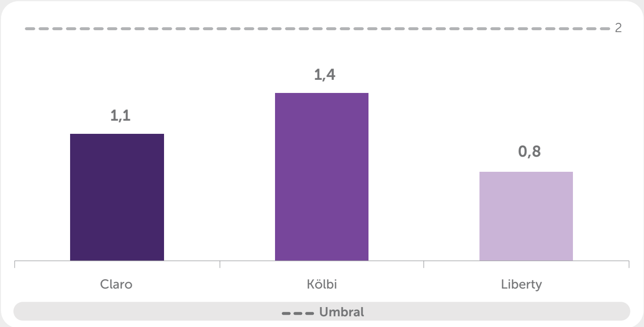
GRÁFICO 4. Porcentaje llamadas interrumpidas en la red 3G, para el año 2025 (Cifras en porcentajes)
