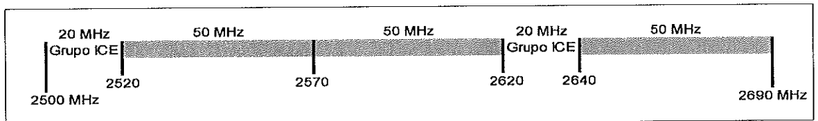
Canalización banda de 2600 MHz
