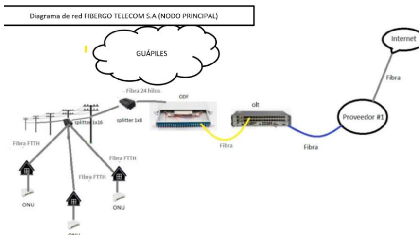
Figura 5. Diagrama de red alámbrica. Aportado por FIBERGO TELECOM S.A.
